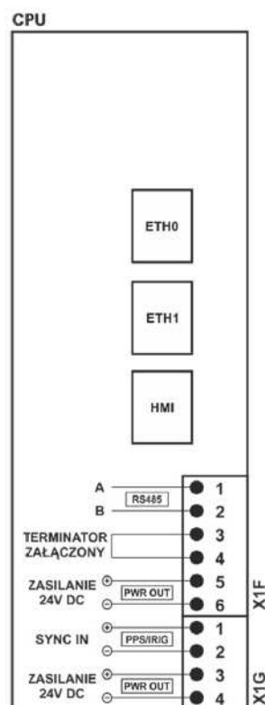
Rys. 1. Widok modułu procesora
